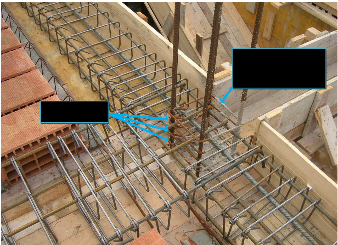
(25) SI – Sono state correttamente inserite le staffe dei pilastri nello spessore del solaio
