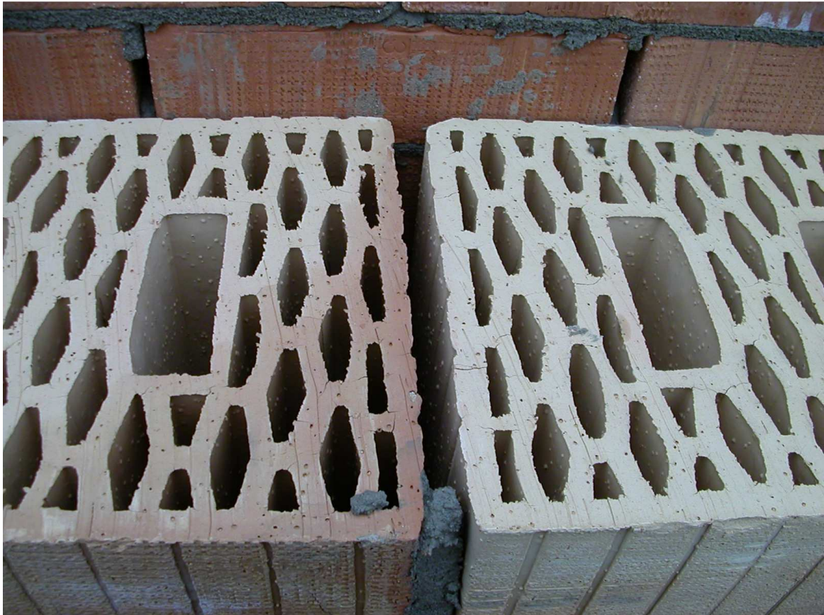
(45) NO – Muratura eseguita praticamente senza giunti verticali di malta
