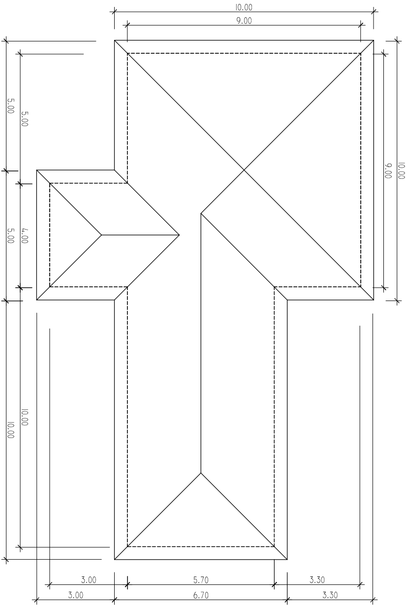
PIANTA
