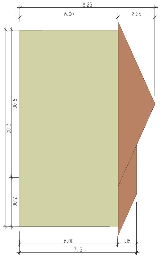
PROSPETTO OVEST
